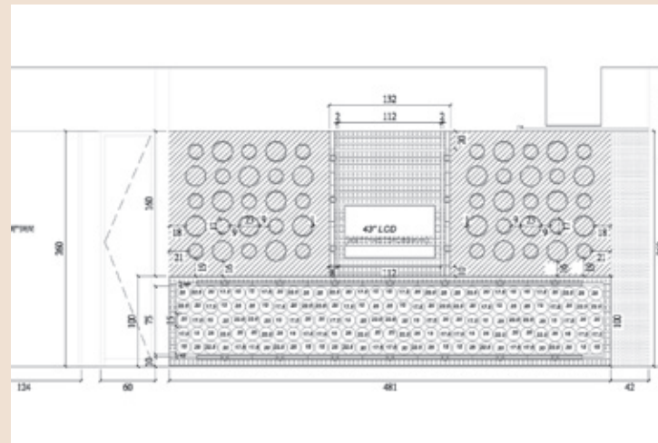
撲克會場 2D施工圖
